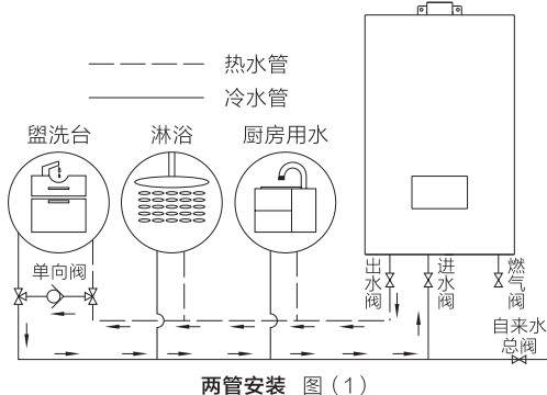
两管安装 图（1）
