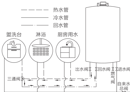
三管安装 图（2）
