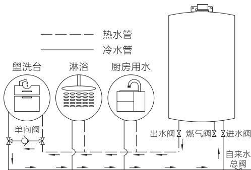
两管安装 图（1）
