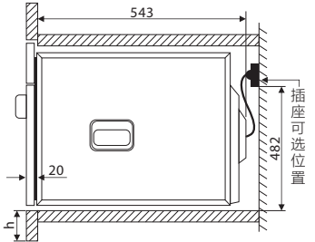
安装侧视图
