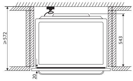
产品俯视图
